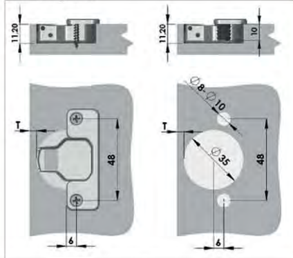
Çanak Ölçüleri
