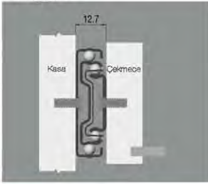
Montaj Şekli
