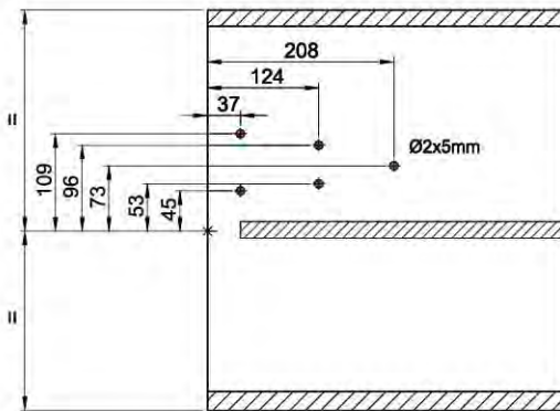
Bağlantı delik merkezleri.
