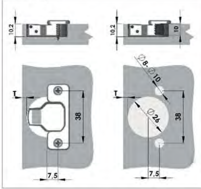
Çanak Ölçüleri
