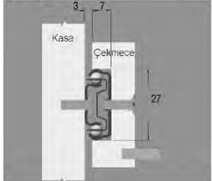
Montaj Şekli
