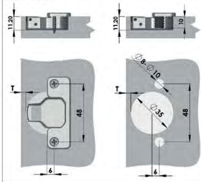
Çanak Ölçüleri
