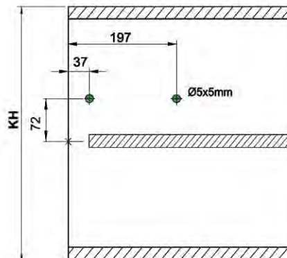
Gövde sabitleme pimi delik merkezleri.
